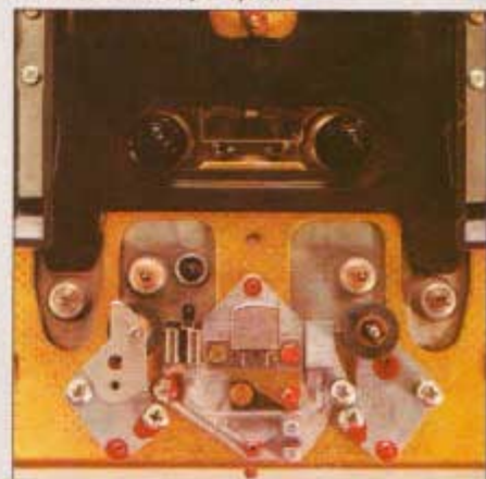
En av de spesielle egenskapene til TCD 310: Bånddriftssystemet med 2 drivaksler/svinghjul og 2 pressvalser i et lukket sløyfex system.
