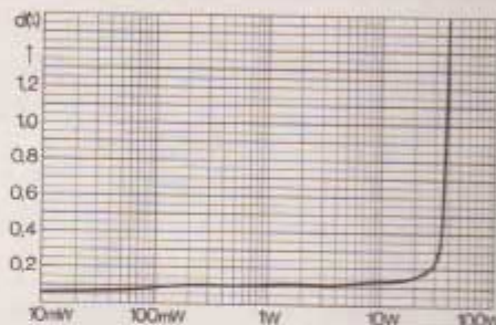
Klirrkurver for lavfrekvensforsterkerne (begge kanaler samtidig) R_L = 4 ohm.
