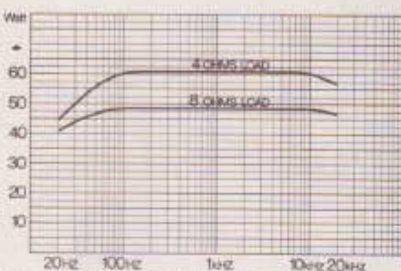
Utgangseffekt som funksjon av frekvens (begge kanaler samtidig, 0,2% klirring).
