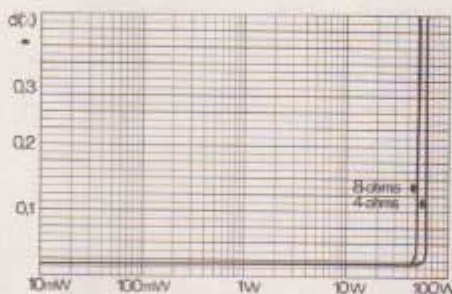
Klirring som funksjon av utgangseffekt (begge kanaler samtidig).
