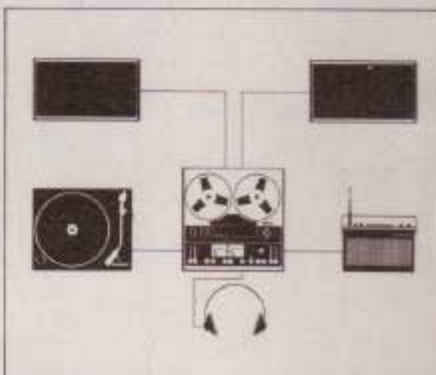
3400X som sentral i et Tandberg Musikknett, tilkopleet 2 stk. Tandberg høyttalere TL 1520, Tandberg Reiseradio TP 41, en platespiller og hodetelefon.
