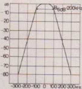
Selektivitetskurve for FM-mottakeren.
