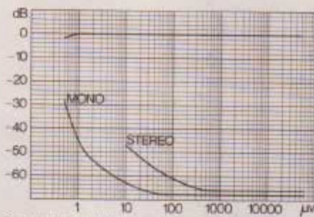
Signal/støyforhold i stereo og mono for FM-delen.
