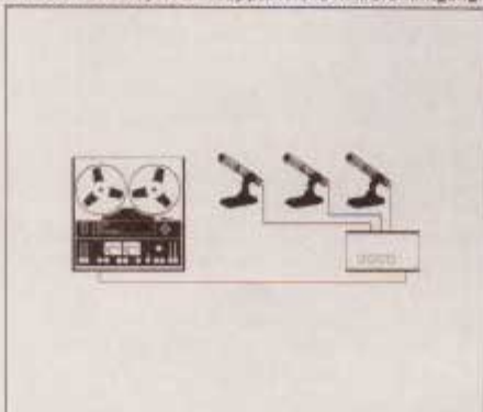
3400X som mikrofonforsterker. Ved forsterking eller opptak av gruppesamtaler benyttes flere mikrofoner som koples til en Tandberg Mikrofonmikser. Mikrofonmikseren er tilkopleet båndopptakerens mikrofoninngang.
